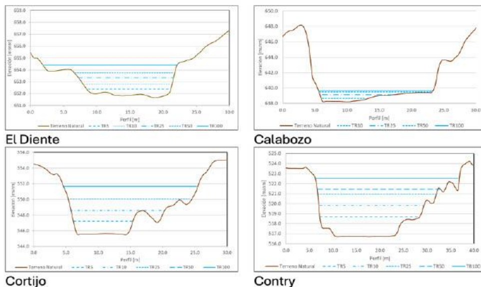
Figura 6. Nivel del río por sitio para diferentes eventos de precipitación con diferentes periodos de retorno.
