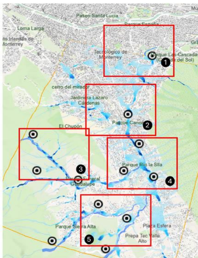
Figura 37. Zonas inundables de acuerdo con la modelación automática del modelo de elevación digital con una precipitación de 60 mm en 1h.
